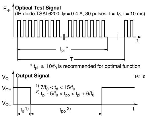
Fig. 1 - Output Function
