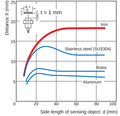
E2E-X18MY
