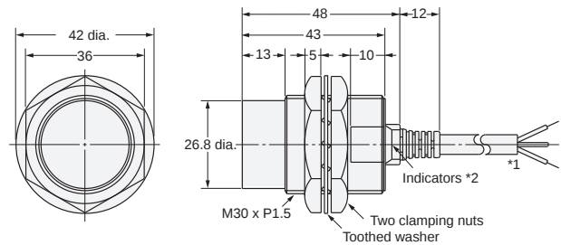
E2E-X20MD1S
