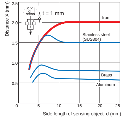
E2E-X2MY
