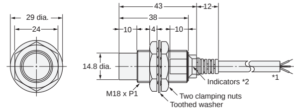
E2E-X14MD1S
