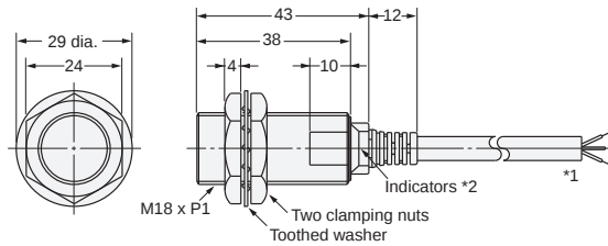
E2E-X7D1S
