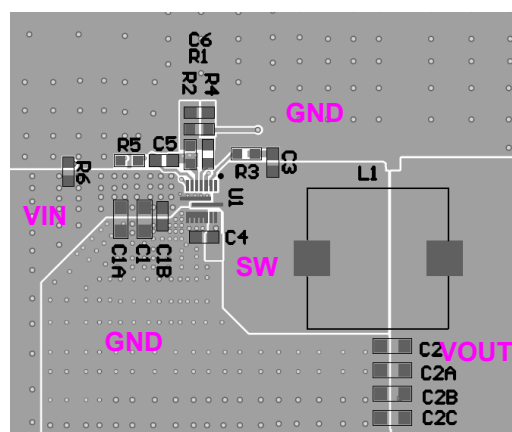
Top Layer
