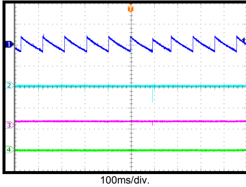
Input/Output Ripple
