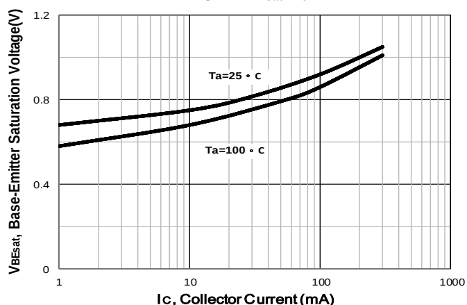
FIG.4 - V_{BEsat} - I_C
