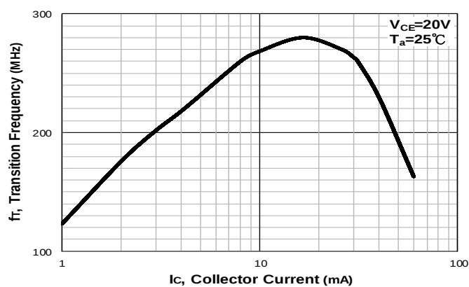
FIG.8 - f_T - I_c
