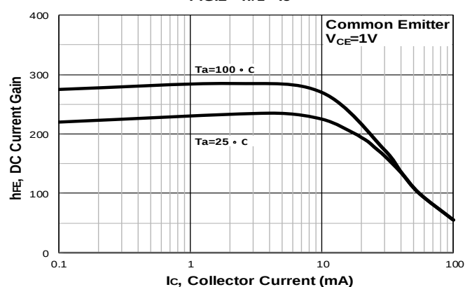
FIG.2 - h_{FE} - I_C
